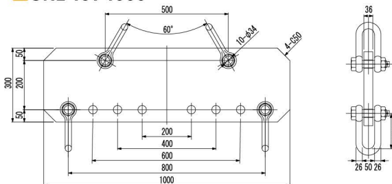
■ ONE-16T-1300 吊り荷重16t 長さ1300mm 本体重量190kg 上下使用ジャックル: RS-10T
