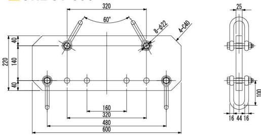
■ ONE-10T-1000 吊り荷重10t 長さ1000mm 本体重量81kg 上下使用ジャックル: RS-8T
